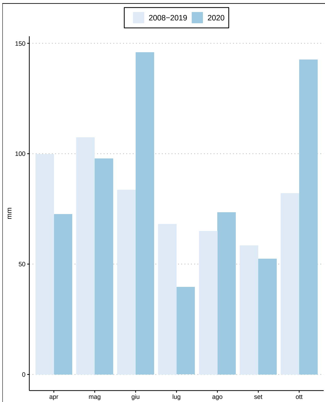
Figura 2: Valori cumulativi mensili di precipitazioni rilevati a Vercelli nel 2020 in confronto con la media delle rilevazioni 2007-2018. Dati CREA-DC in confronto a dati telerilevamento NASA.
